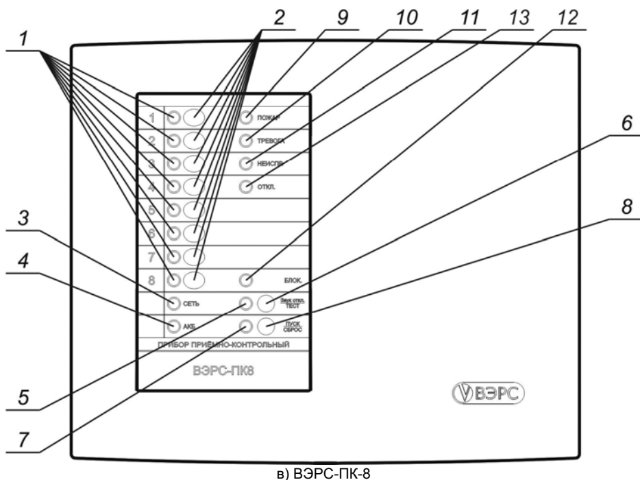
Рисунок А1. Внешний вид передней панели приборов ВЭРС-ПК(8,4,2)(П,М)(Т)(LAN) Версия 3.2.
