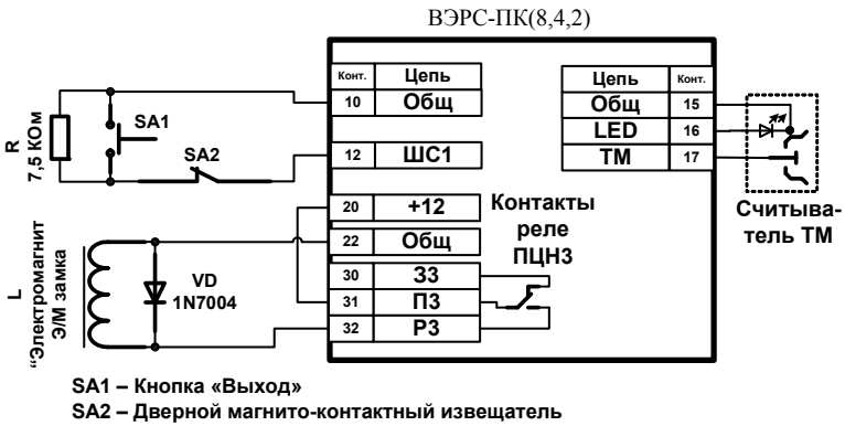
Рисунок Б3. Схема организации Точки доступа.
