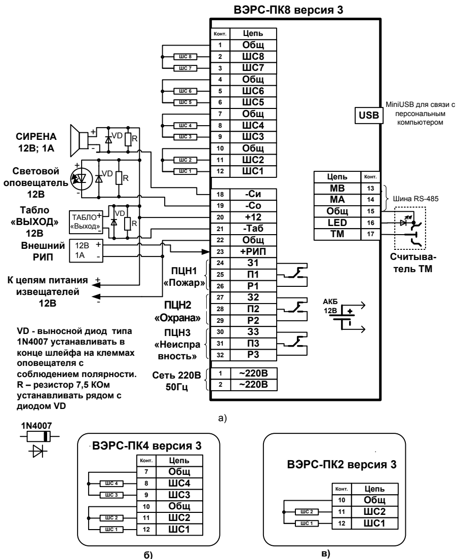
Рисунок Б1. Схемы внешних соединений приборов ВЭРС-ПК(8,4,2) версия 3.2.
