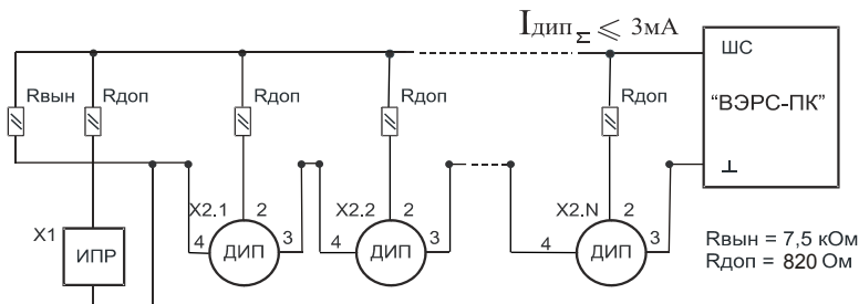
Рисунок.Б4. Схемы включения ШС типа ШННС и ШПНС с несколькими дымовыми извещателями (типа ИП212). Двухпороговый алгоритм с верификацией.
