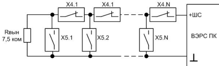
Рисунок Б8. Схема включения охранных извещателей в ШСО.
