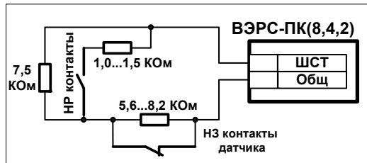
Рисунок Б9. Схема включения технологических датчиков в ШСТ.
