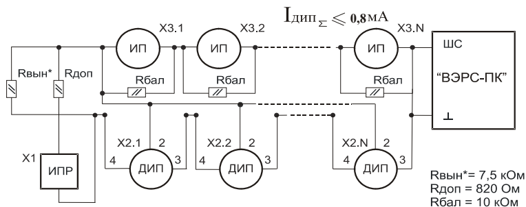
Рисунок.Б5. Схемы включения ШС с несколькими тепловыми извещателями (типа ИП-105). Двухпороговый алгоритм с верификацией.
