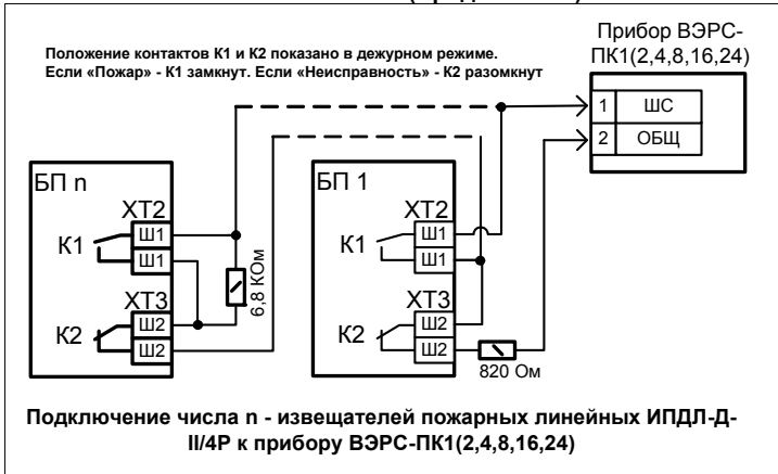
Рисунок Б7. Схема включения линейных дымовых извещателей ИПДЛ-Д-II/4Р.
