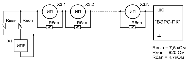
Рисунок.Б5. Схемы включения ШС с несколькими тепловыми извещателями (типа ИП-105). Двухпороговый алгоритм с верификацией.
